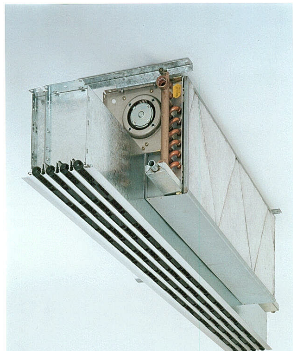
Ventilatorconvector Typ LVC
