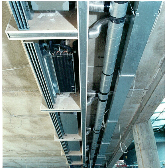
Installatievoorbeeld: Inductieunit, type: LHG
